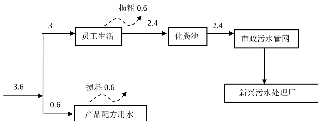
图 2-2 项目水平衡图（单位：m³/d）
