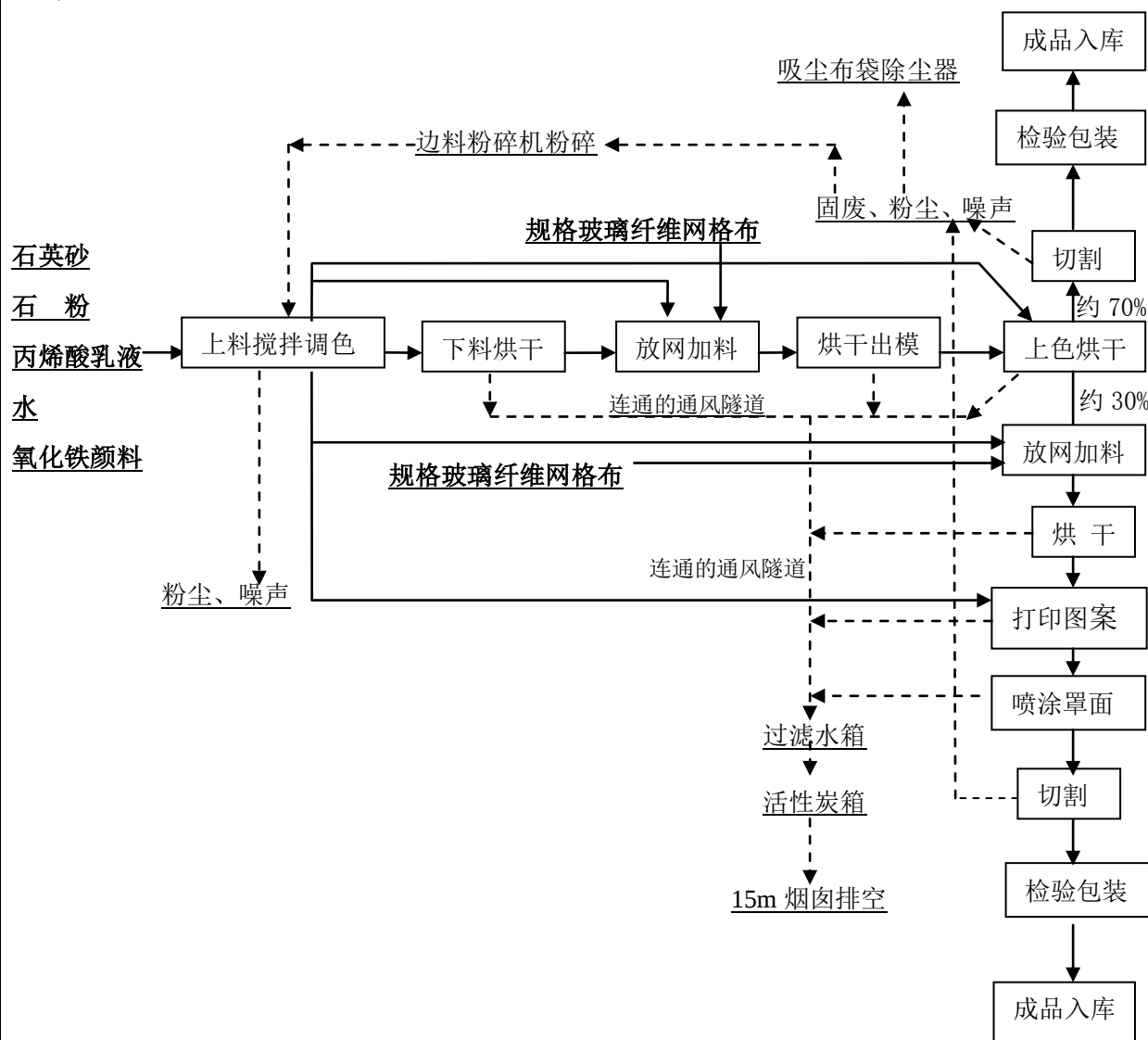
图 2-1 建筑新型轻质软瓷砖生产线工艺及其排污节点图
