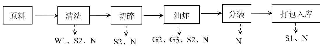
图 2-4 辣椒油调味品工艺流程及产污环节图
