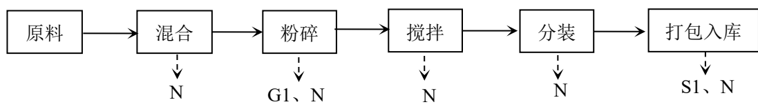
图 2-2 项目汤料包调味品生产工艺流程及产污环节图
