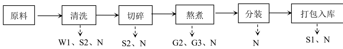
图2-3 项目酱料包调味品生产工艺流程及产污环节图
