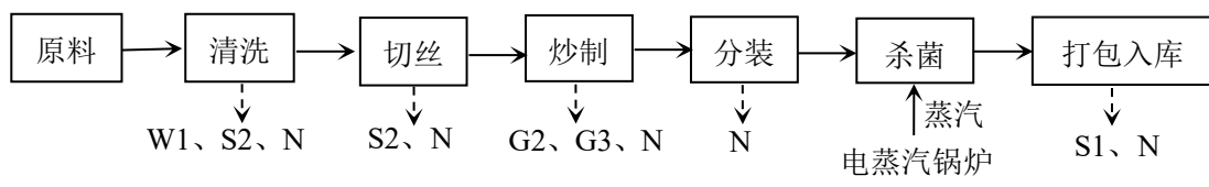
图 2-5 酱腌菜工艺流程及产污环节图
